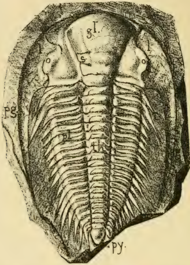
Fig. 376. — Paradoxides . 1 er lobe : Tête, gl , glabella; s , s , sillons latéraux de la glabella; l , limbe; o , œil (certains genres en sont dépourvus); pg , pointes génales (manquant dans certaines formes). 2 e lobe : Thorax. th , segments thoraciques; pl , plèvres (ici du type dit : plèvres à sillons). 3 e lobe : Pygidium, pg , pygidium (uni ici, il est quelquefois sillonné).
